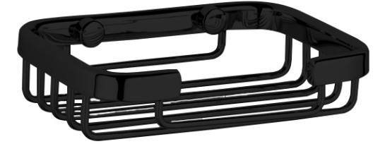
065101-N ● ● Esponjera rejilla rectangular pequeña. Acabado: negro mate. Material: latón. Small square shower basket grid. Finish: matte black. Material: brass. 35 x 132 x 95 mm.
