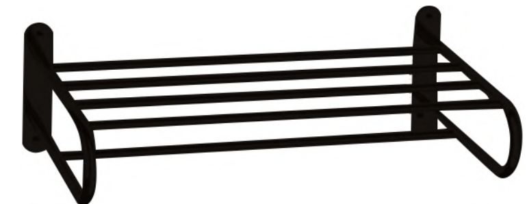
061500-N ●●●●● Toallero repisa pletinas con barra 4 anclajes 50 cm. Acabado: negro mate. Material: latón. Towel shelf with bar and 4 anchors 50 cm. Finish: matte black. Material: brass. 145 x 480 x 260 mm.
