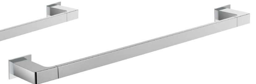
161401 ● ● Toallero barra 50 cm KUO ADHESIVO. Acabado: cromo brillo. Material: latón. Towel bar KUO ADHESIVE 50 cm. Finish: bright chrome. Material: brass. 43 x 518 x 74 mm.
