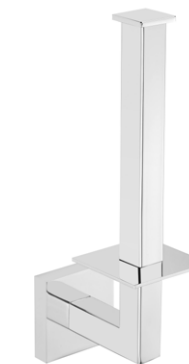
110500 ●●○ Portarrollos reserva AVANT. Acabado: cromo brillo. Material: latón. Reserva toilet roll holder AVANT. Finish: bright chrome. Material: brass. 195 x 50 x 85 mm.
