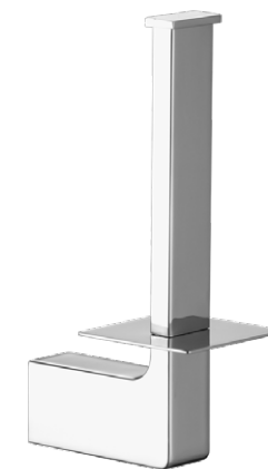
160101 ●●●●● Portarrollos reserva KUO. Acabado: cromo brillo. Material: latón. Reserva toilet roll holder KUO. Finish: bright chrome. Material: brass. 169 x 55 x 94 mm.
